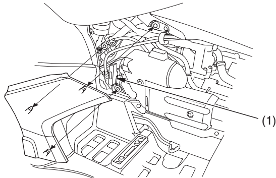
(1) käsi käynnistin
