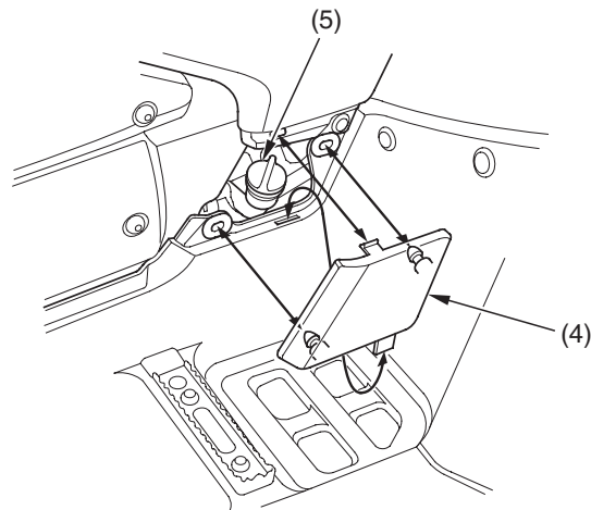
(4) öljyn täyttökorkin kansi
