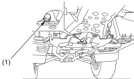
(1) moottoriöljyn tyhjennystulppa
