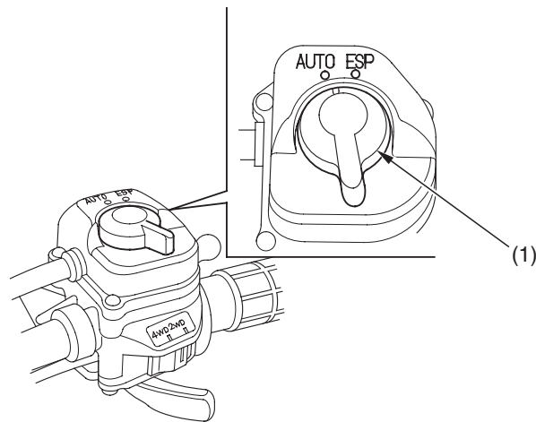
(1) vaihteiston valintakytkin
