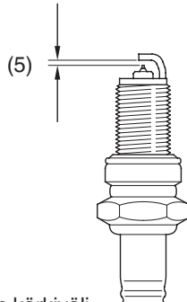
(5) sytytystulpan kärkiväli
